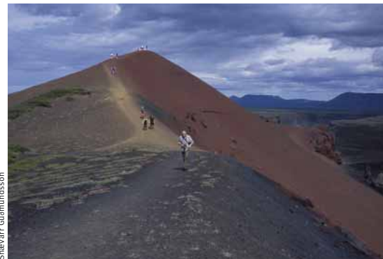
Rauðhólar formationer, en del af en gammel række af kratere.
